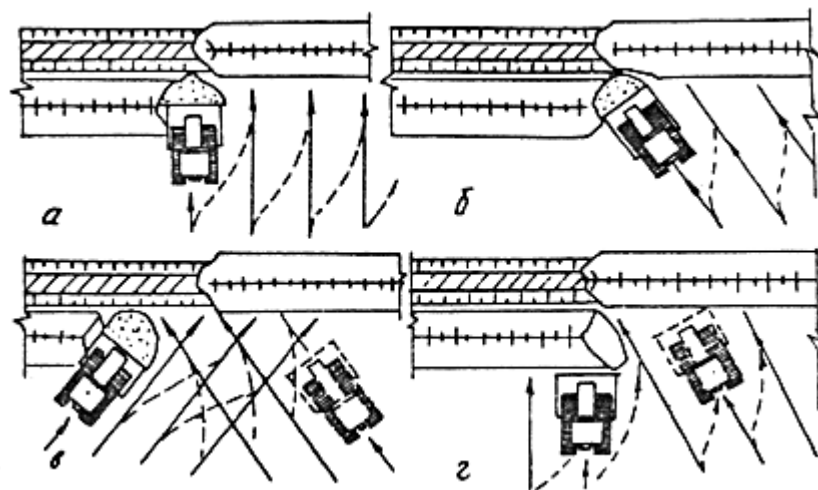
Рис. 7. Схемы производства работ по засыпке уложенного трубопровода бульдозером: а - прямолинейными проходами; б - косопоперечными параллельными проходами; в - косопоперечными параллельными проходами; г - комбинированным способом
